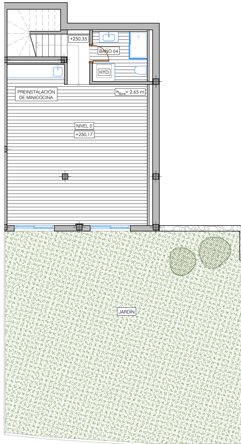
NIVEL 0
