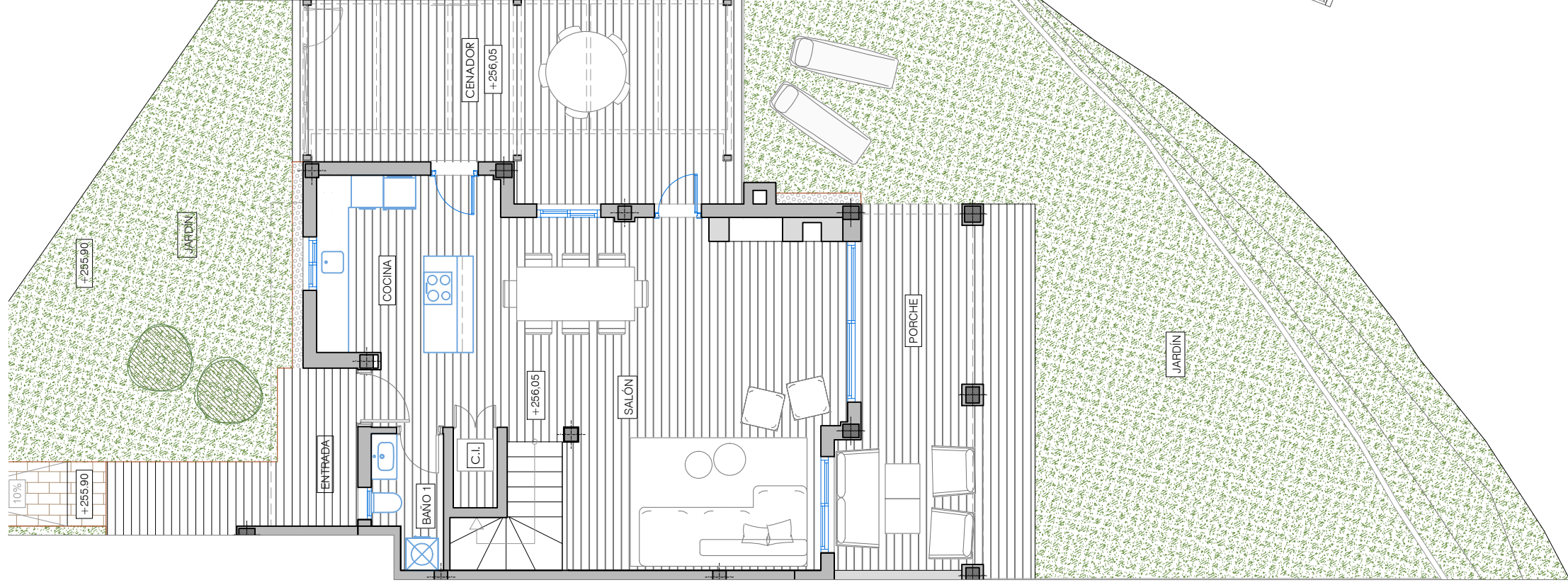
NIVEL 1
